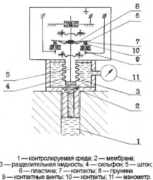
Схема принципиальная кинематическая и электрическая реле РД-314РМ с нормально замкнутыми контактами
