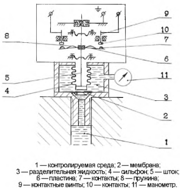
Схема принципиальная кинематическая и электрическая реле РД-314РМ с нормально разомкнутыми контактами
