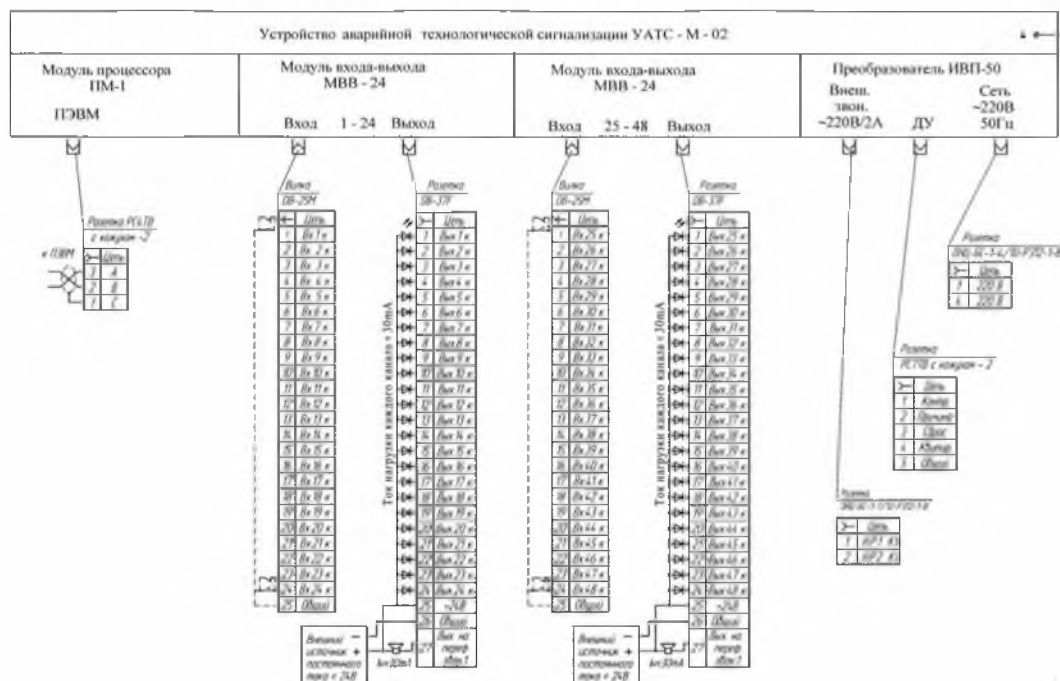
Схема внешних соединений устройства УАТС-М-02
